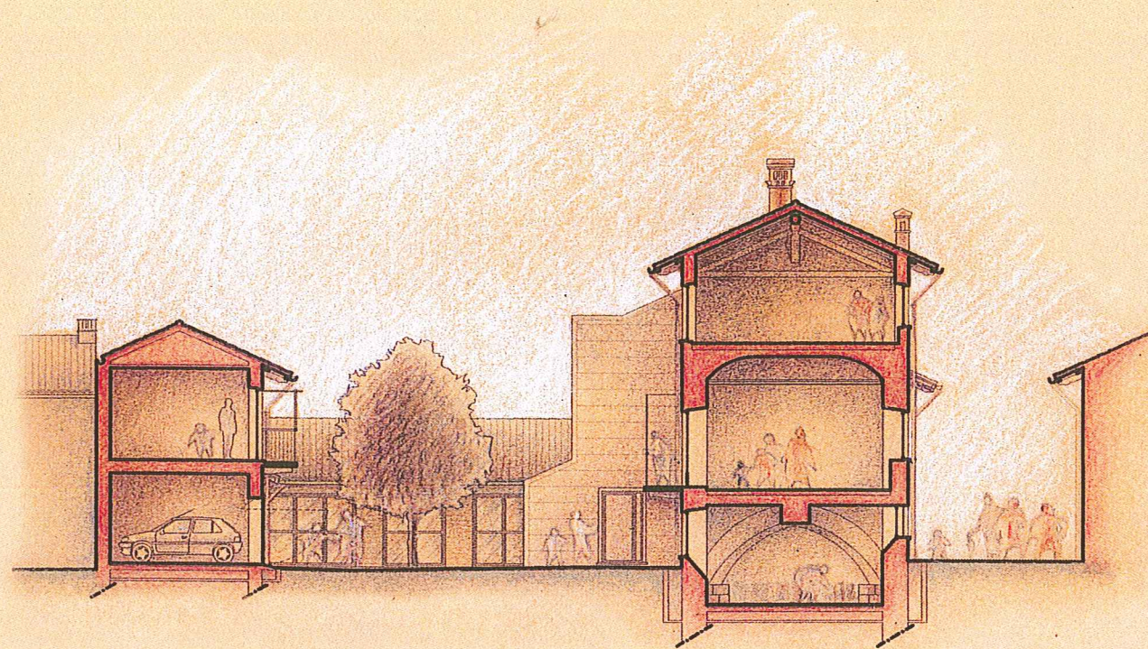
SEZIONE B-B SCALA 1:200 \frac{1}{0} \text{---} 6 \text{m}
